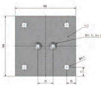
ПЛАСТИНА - MVA 400 W
