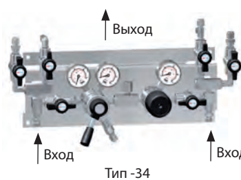
Тип -34 (с продувкой инертным газом)
