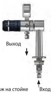
Подвесное исполнение вход сверху (исполнение HW)
