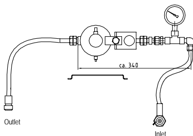
Пример: однобаллонная система с контактными манометрами
