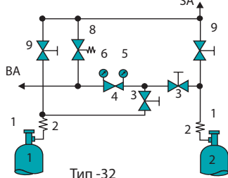
Тип -32 (с вентиляционным трубопроводом)
