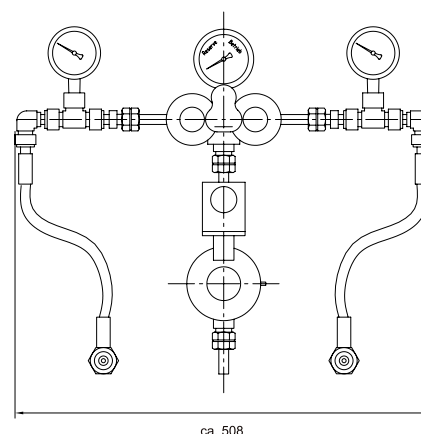
Пример: двухбаллонная система с контактными манометрами
